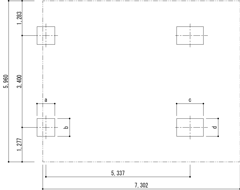
■ 基礎配置図
